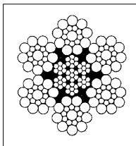
IWRC 6×S(19)
