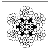
IWRC 6×WS(26)
