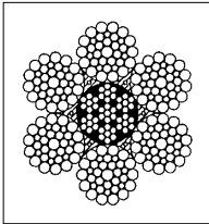
デルタフィラーロープ DF IWRC 6×WS(36)
