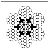
IWRC 6×W(19)
