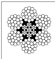
IWRC 6×Fi(25)
