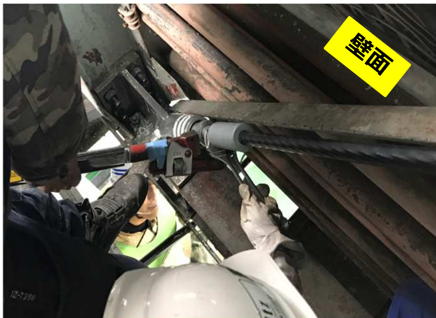
トルクレンチでの張力導入状況
